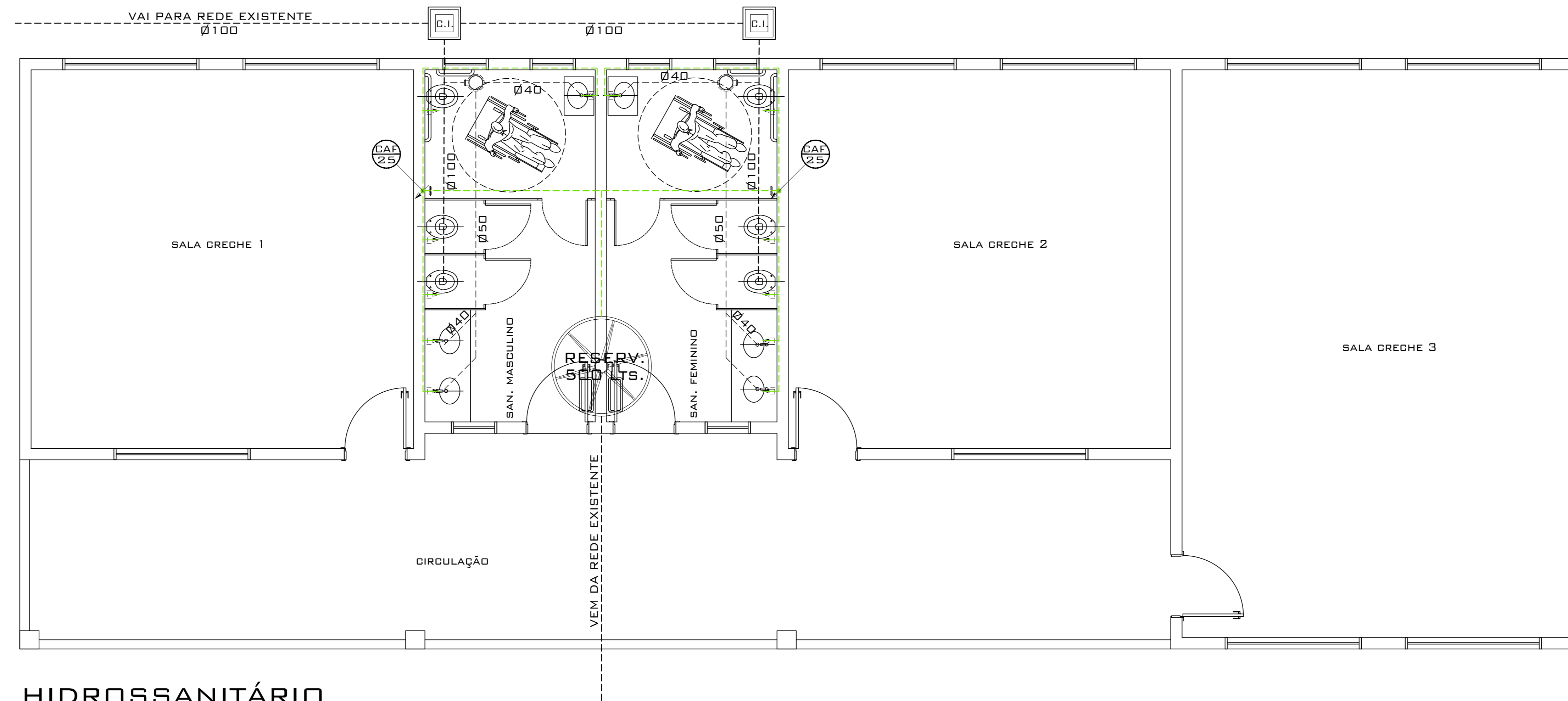
HIDROSSANITÁRIO ESC.: 1/50
