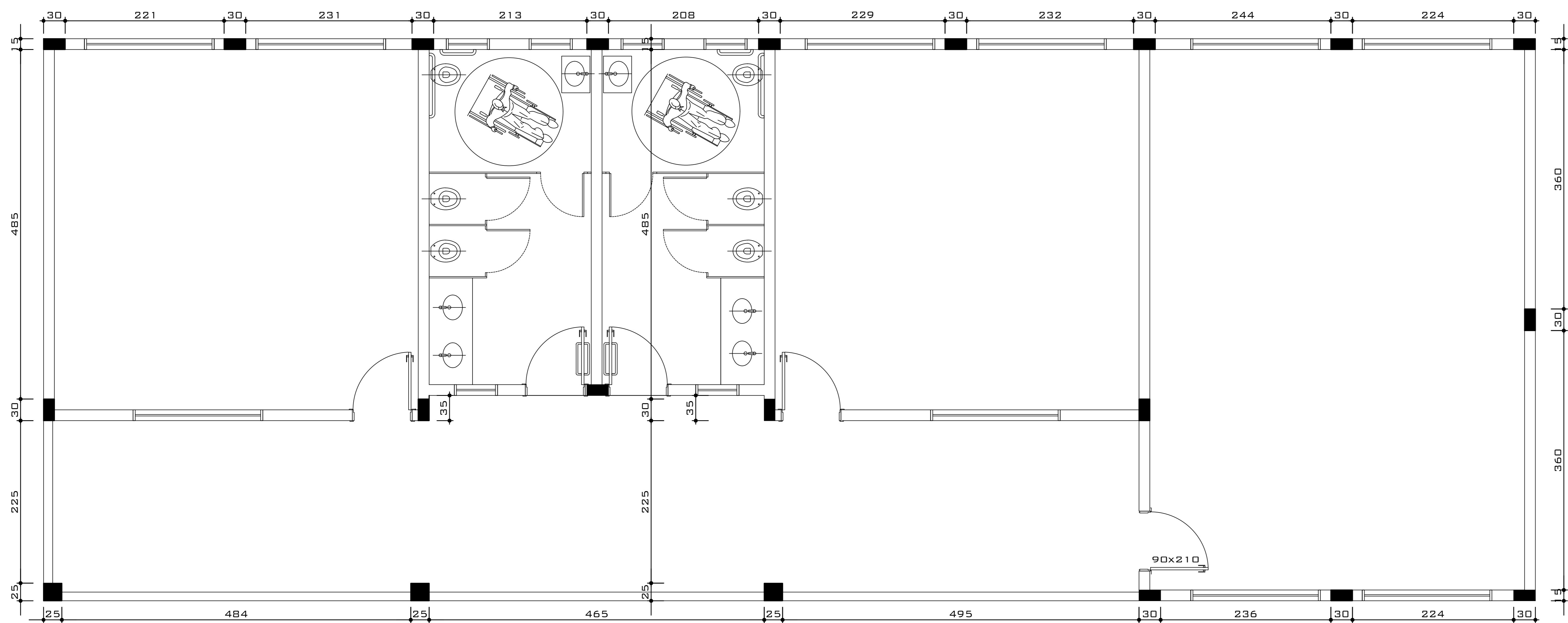
PLANTA BAIXA ESTRUTURAL ESC.: 1/50 ÁREA.: 161,46 M 2
