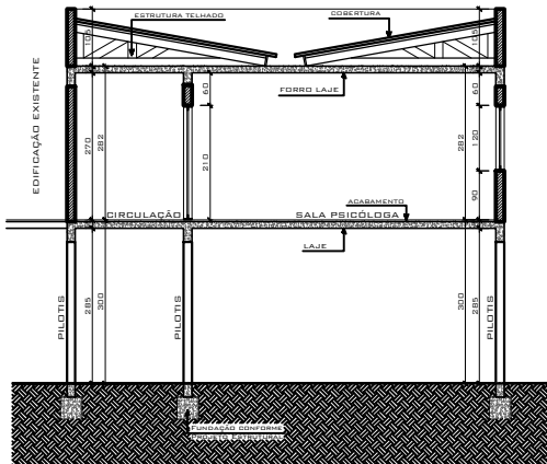
CORTE A-A ESC.: 1:50
