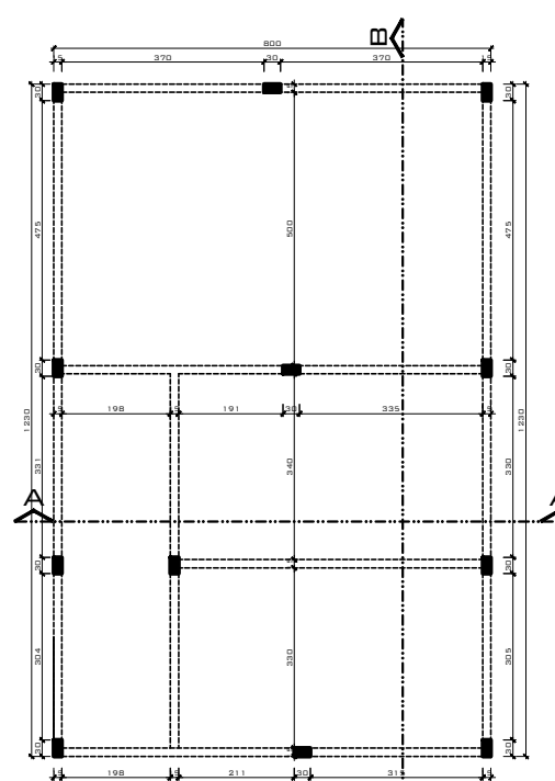
PLANTA BAIXA PILOTTIS ESC.: 1/50
