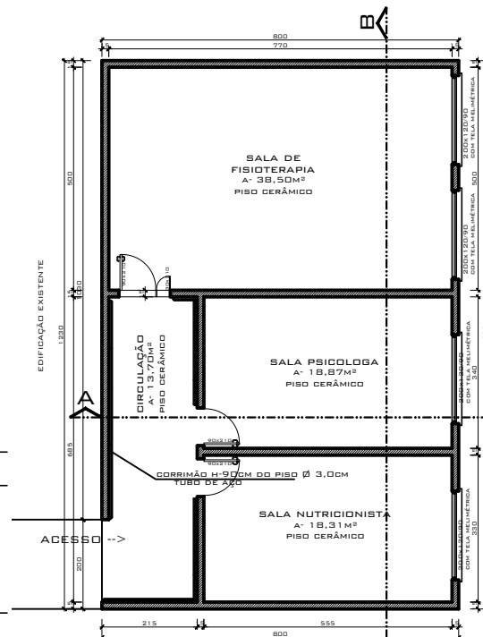
PLANTA BAIXA SUPERIOR ESC.: 1/50 ÁREA: 98,40 M 2
